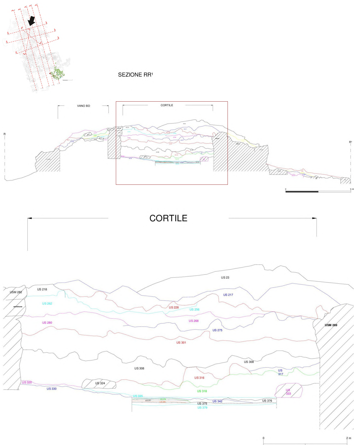
Fig. 51 - SANTADI (SU) - Loc. Pani Loriga. Acropoli scavo 2023-2024. Sezione RR e dettaglio del cortile (rilievo ed elaborazione Vincenzo Nubile)
