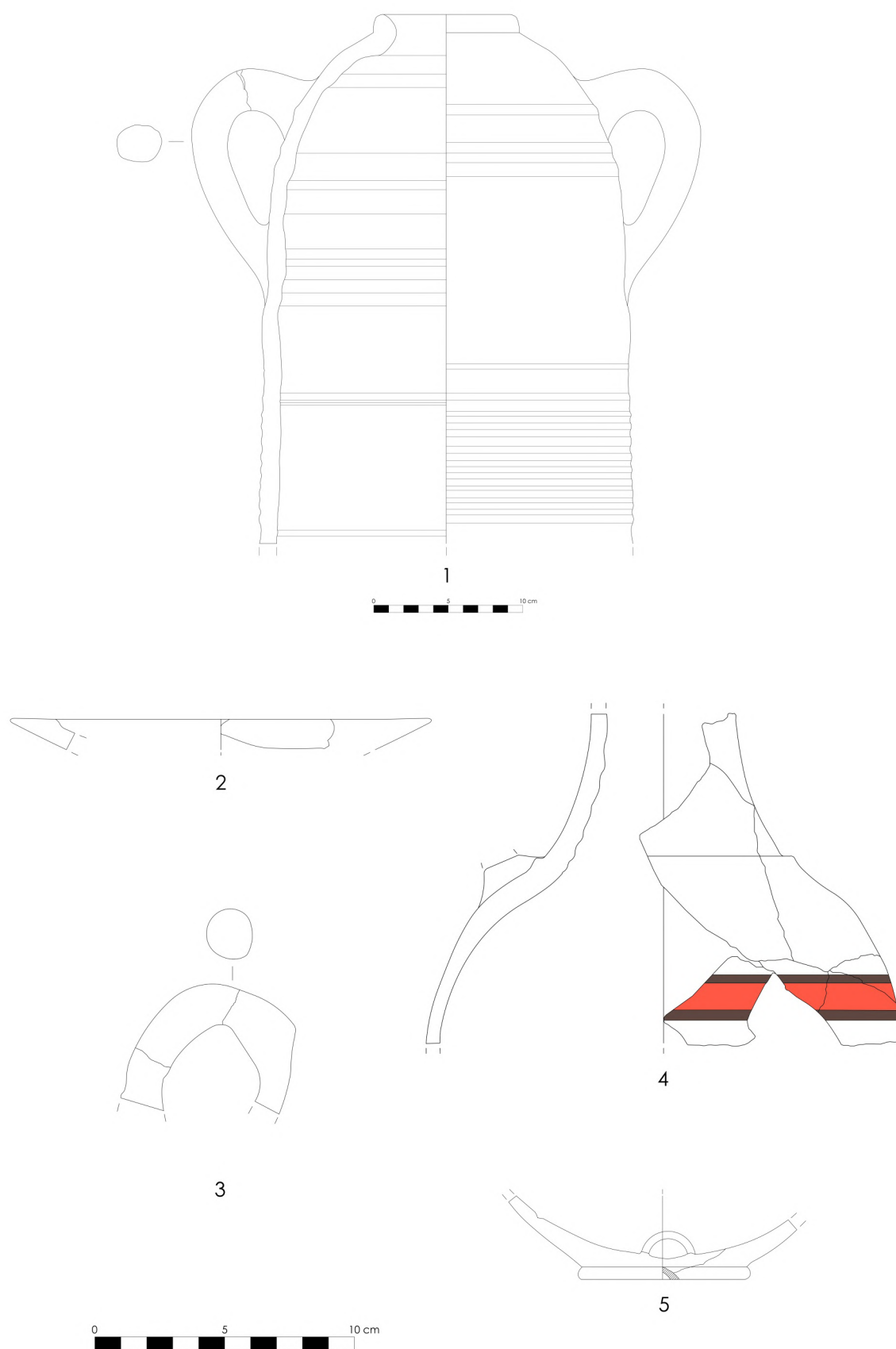
Fig. 30 - SANTADI (SU) - Loc. Pani Loriga. Acropoli scavo 2023-2024. Cortile IM: i materiali. 1: anfora T.1.2.1.2/D2; 2: lucerna; 3: frammento di brocca bilobata o attingitoio; 4-5: brocca bilobata (disegni Marco Matta)
