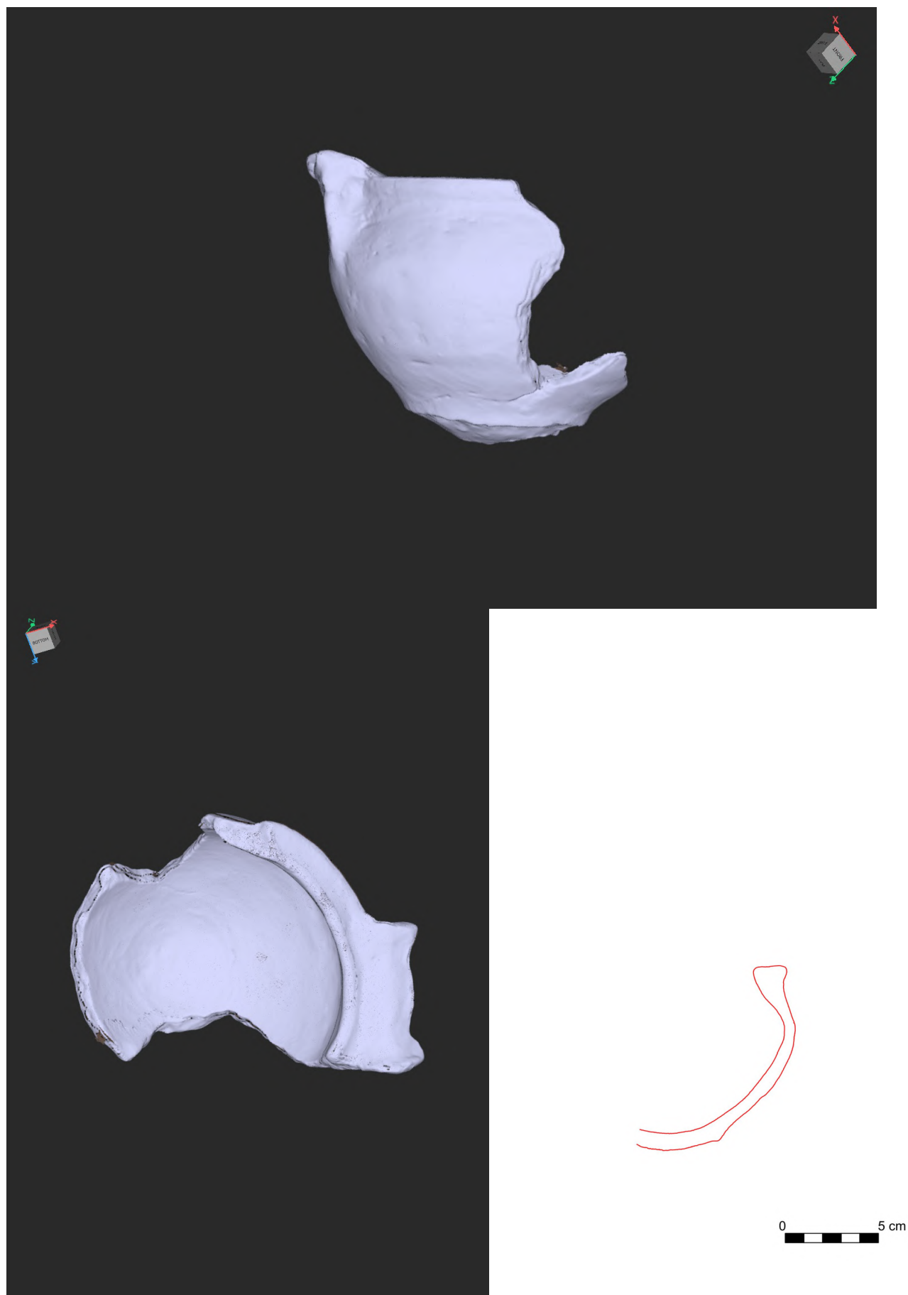
Fig. 14 - SANTADI (SU) - Loc. Pani Loriga. Acropoli scavo 2023-2024. Il recipiente US 296 (rilievo e disegno Pietro Francesco Serreli)
